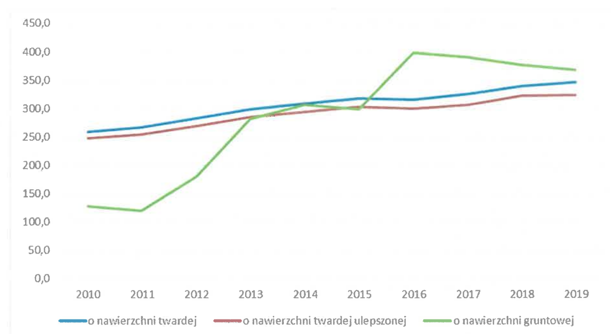
WYKRES 10. KILOMETRY DRÓG WEDŁUG RODZAJU NAWIERZCHNI NA PRZESTRZENI LAT 2010-2019.
